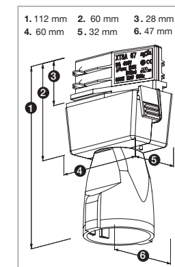
Schuko adapter 16A Adattore Schuko 16A
