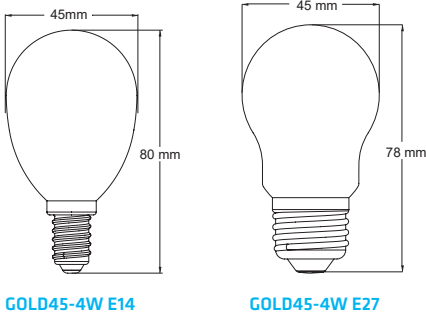
GOLD45-4W E14 GOLD45-4W E27
