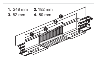
Flexible coupler Giunto di unione flessibil
