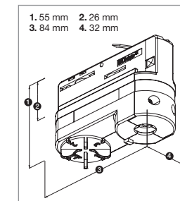
10A Multi-circuit adapter Connection with screw Adattatore multi-circuito 10A Connessione con vite
