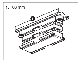
Inner coupler Giunto di unione interno
