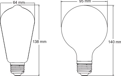
GOLD64-6W E27 GOLD95-6W E27
